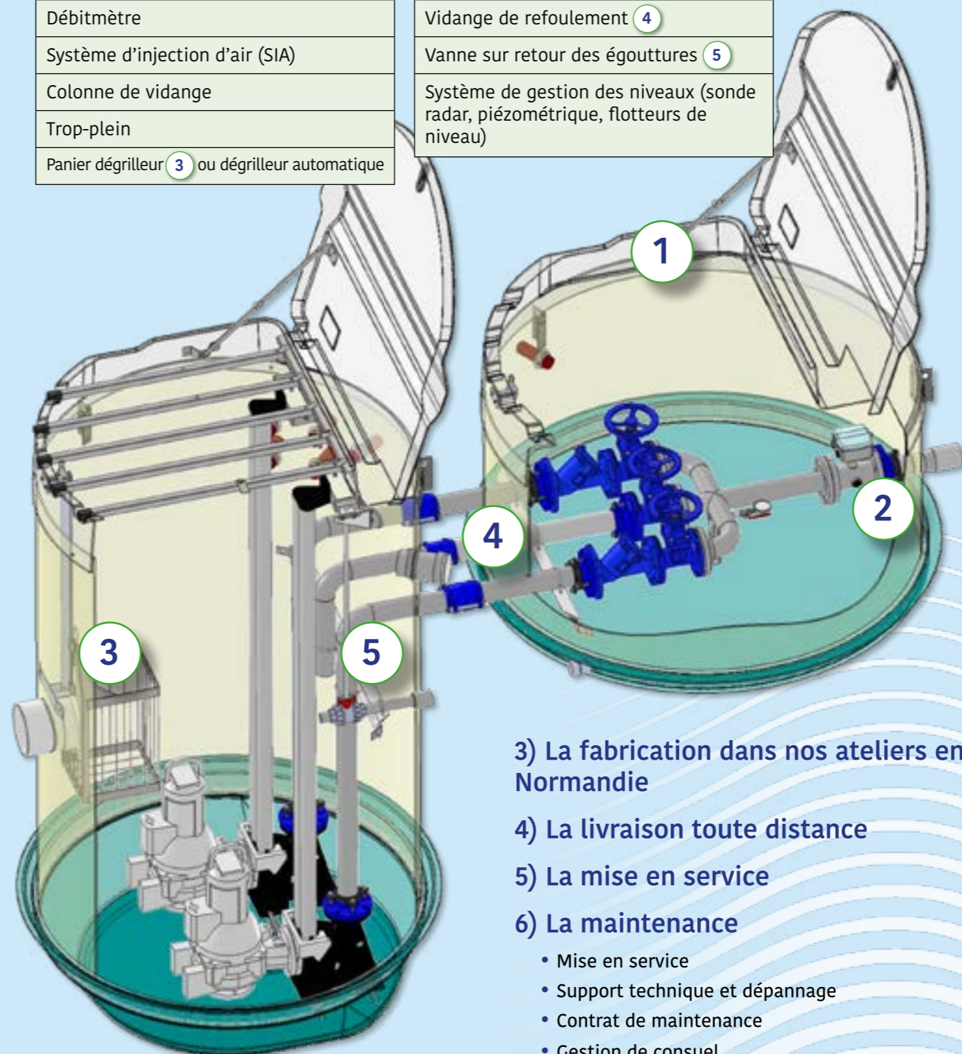
Exemple d'une station de relevage sur-mesure tuyauterie inox (option)
