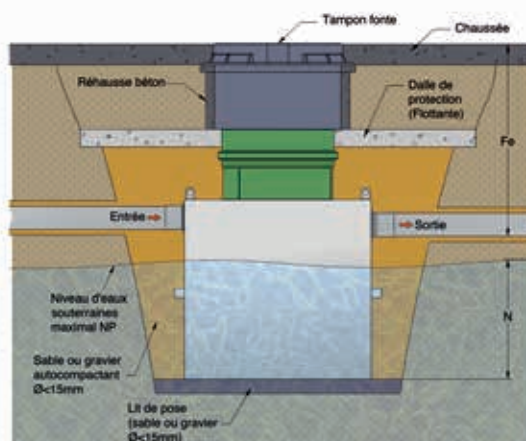
Pose sous voirie
