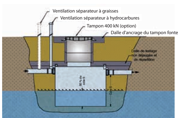
Pose gamme A en présence d'eau souterraine.
