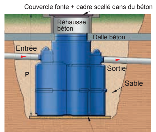
Lit de sable 5 à 10 cm
