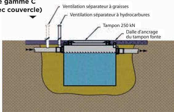
Pose gamme A (Avec amorce)
