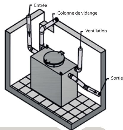
Pose gamme A en présence d'eau souterraine.
