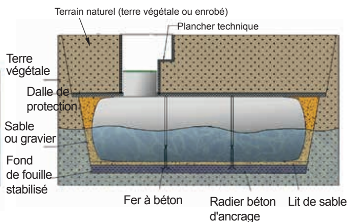
Pose sous dalle de protection
