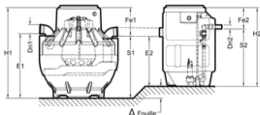
Séparateur hydrocarbures
