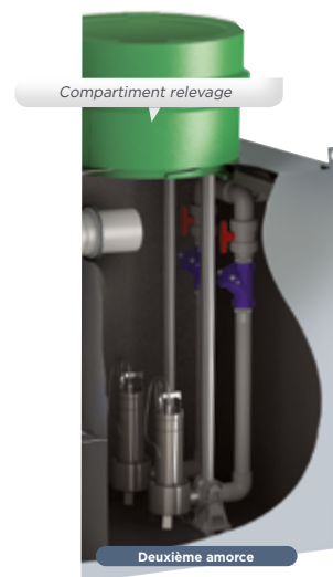
Compartiment relevage réf. Kit KP26P (en option)
