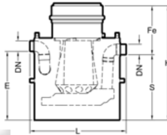
Détail de l'intérieur de l'appareil
