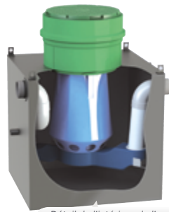
Détail de l'intérieur de l'appareil
